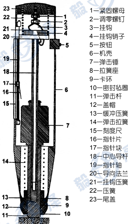
图1 回弹仪构造和主要零件名称
